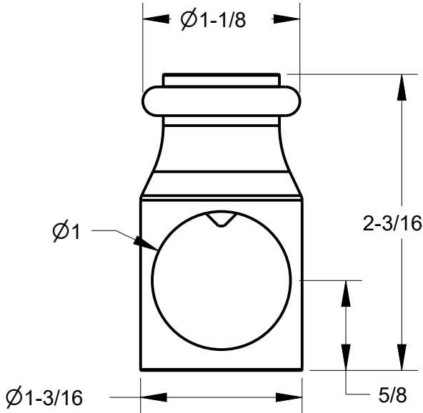
DOOR STOP
