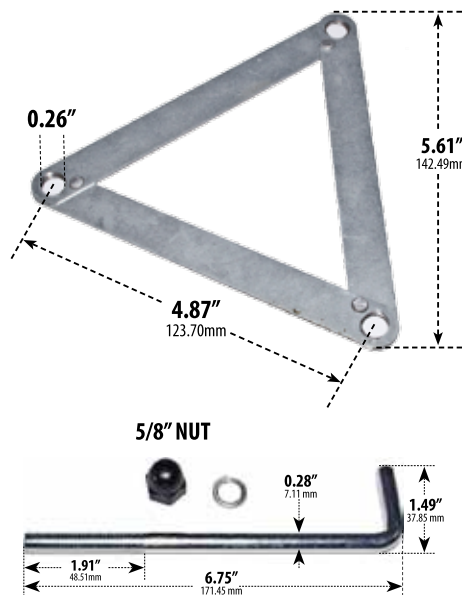
TEMPLATE PATTERN
