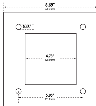
TEMPLATE PATTERN
