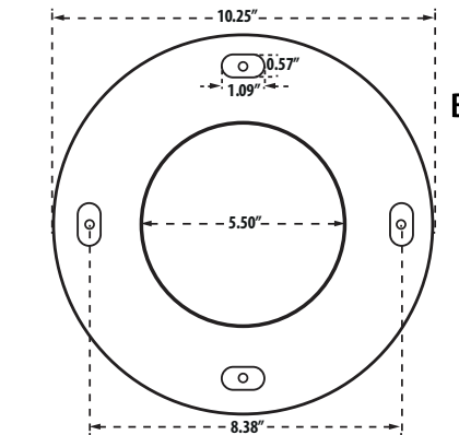
BOLT
